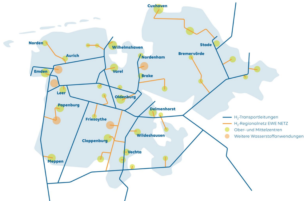
Abbildung 34: Lokale Versorgung des Wasserstoffs
